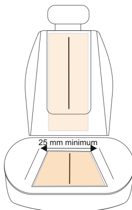
Sitz mit Längsbespannung
